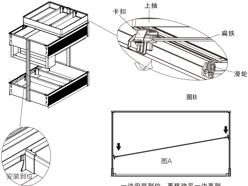
图A 图B 一边安装到位，再移动另一边直到两边水平，滑块到槽内安装到位
