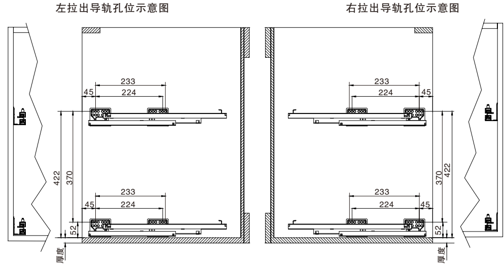
150柜/200柜/250柜侧拉篮导轨安装示意图
